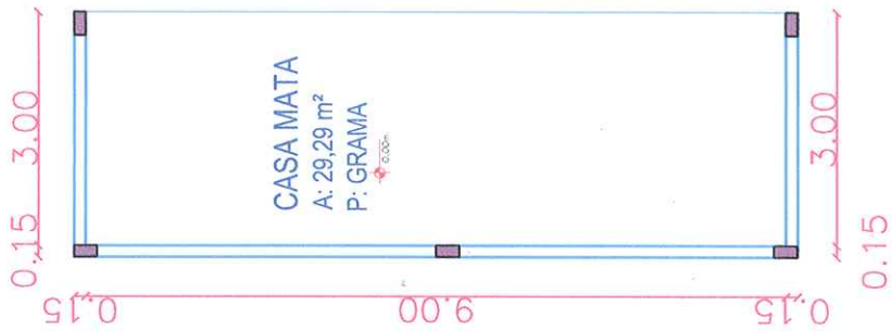
PLANTA BAIXA TÉCNICA CASA MATA Esc:1:75
