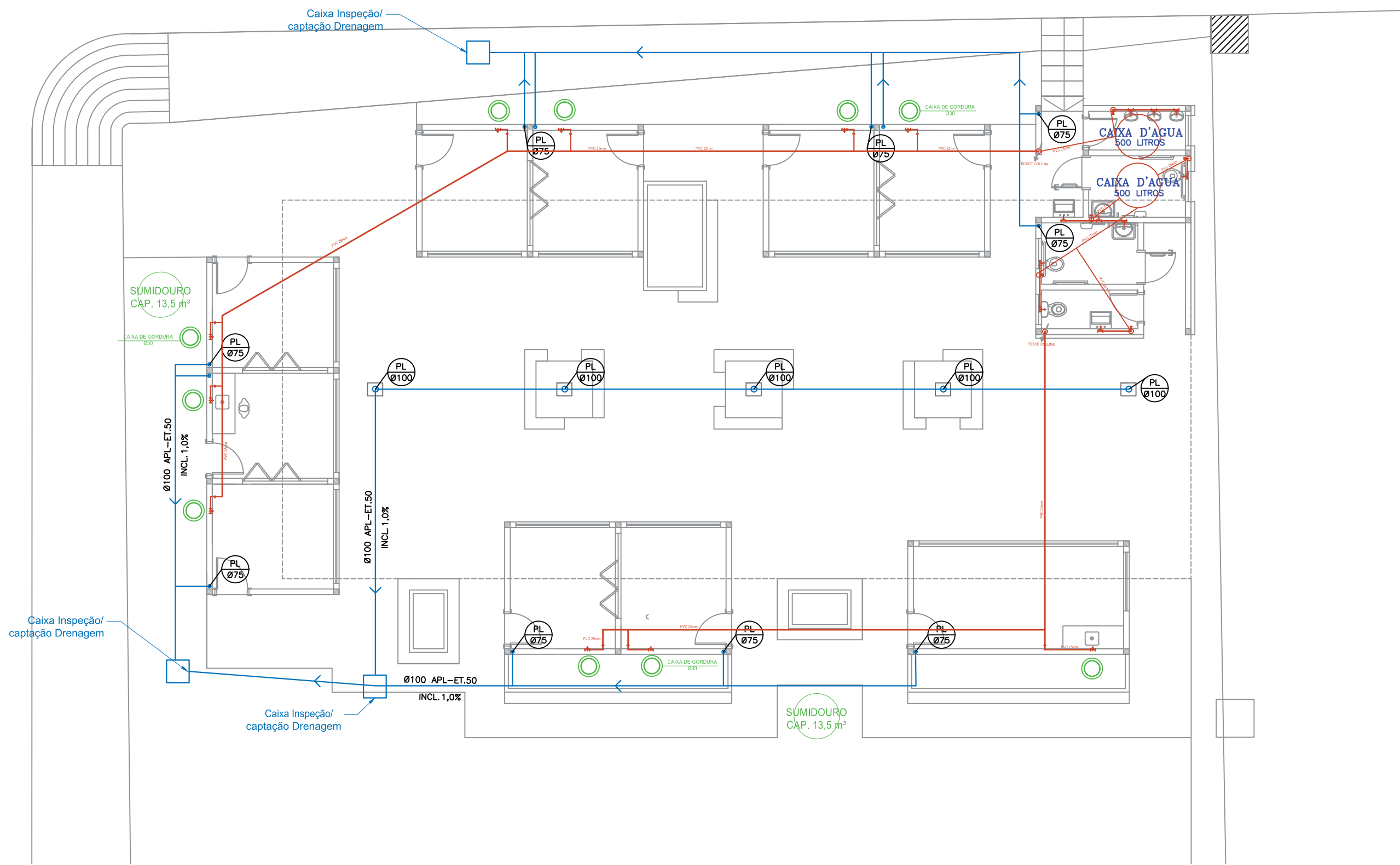
PLANTA HIDROSSANITÁRIO Escala 1|100
