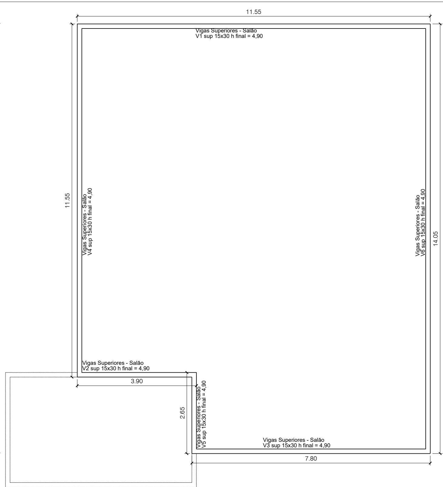
Planta de Forma - Vigas Superiores Salão Escala 1/75
