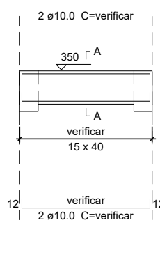
Detalhamento Vigas Sem Escala
