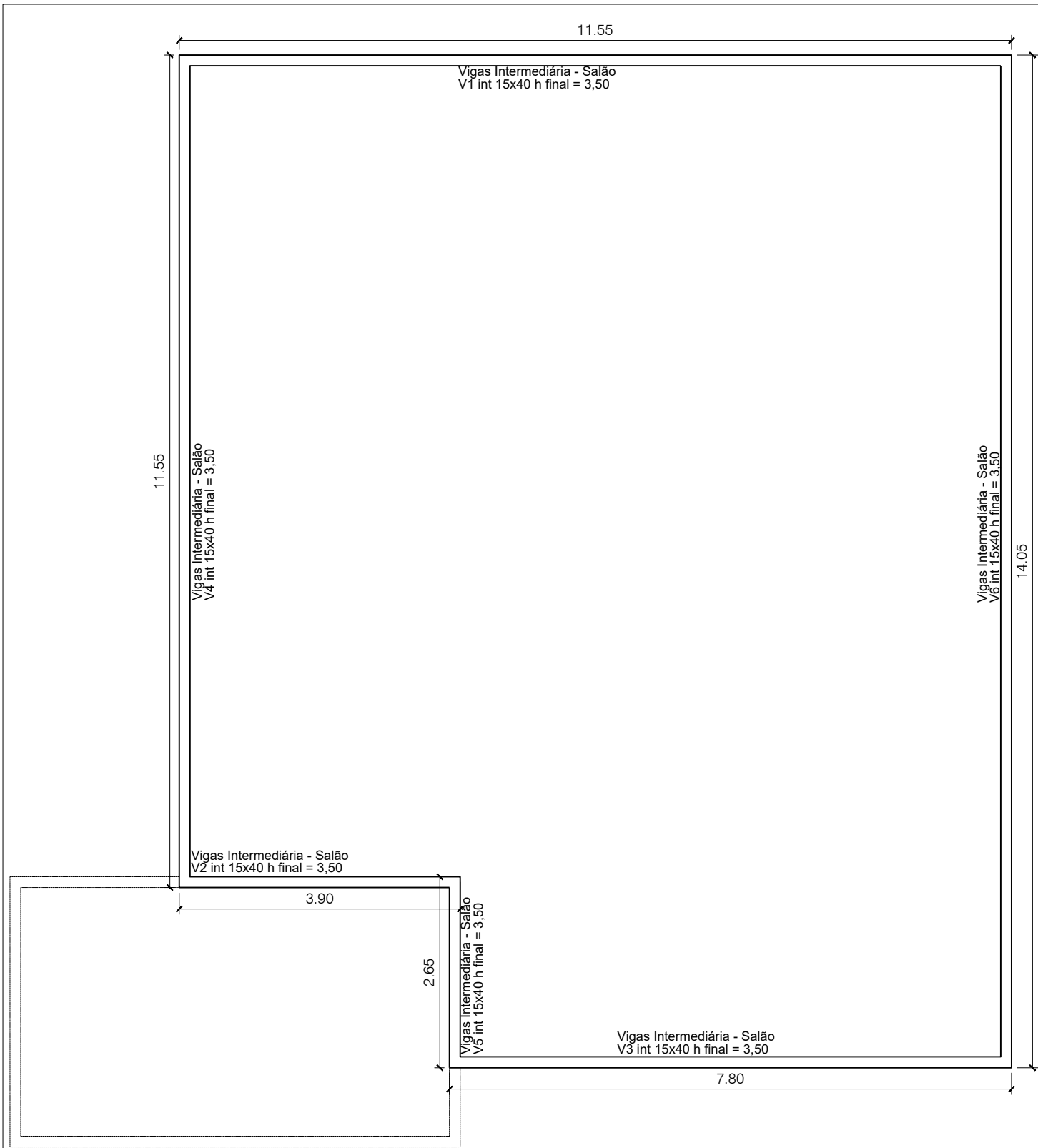
Planta de Forma - Vigas Intermediárias Salão Escala 1/75
