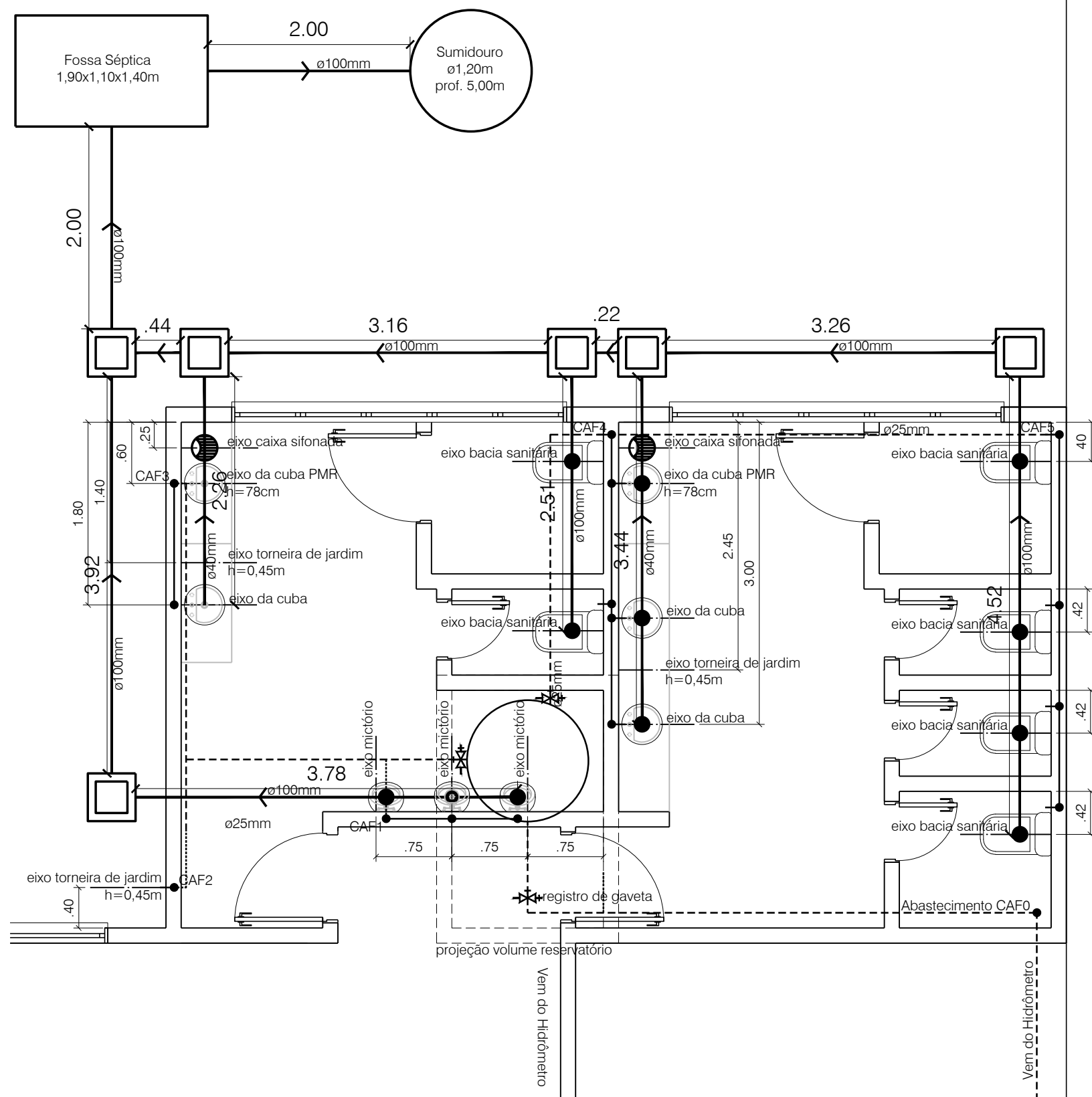
Planta Baixa Hidrossanitário Escala 1/50
